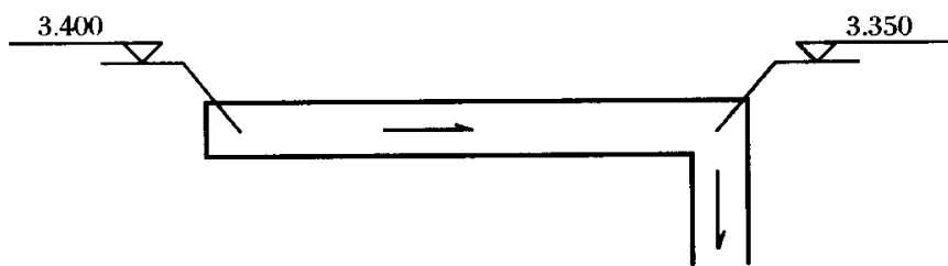
图 2.3.5-2 平面图中沟渠标高标注法
